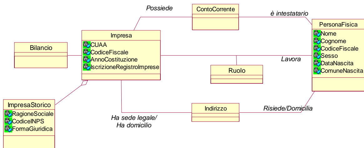
FIGURA 10 – DIAGRAMMA DELLE CLASSI PER IMPRESA E PERSONAFISICA
