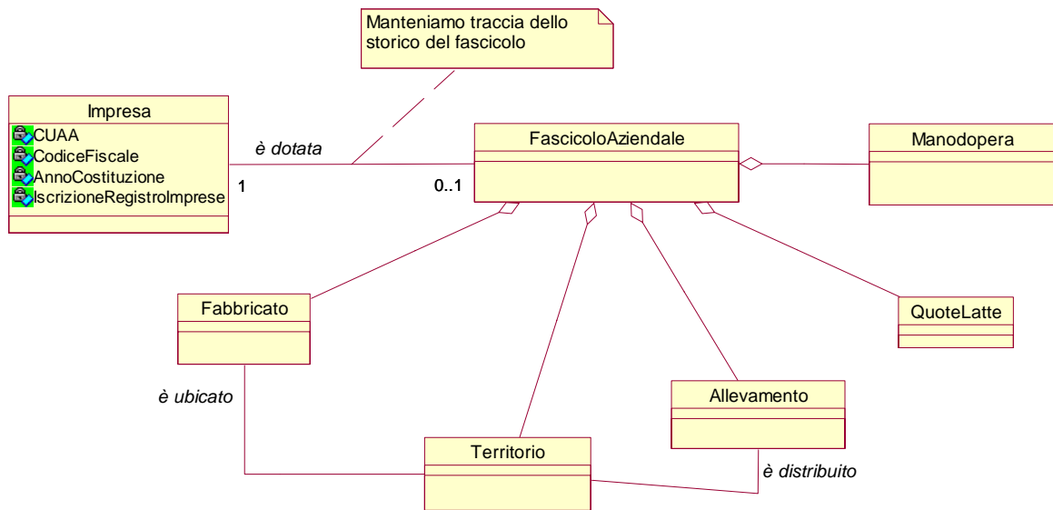
FIGURA 9 – DIAGRAMMA DELLE CLASSI PER IL FASCICOLO AZIENDALE
