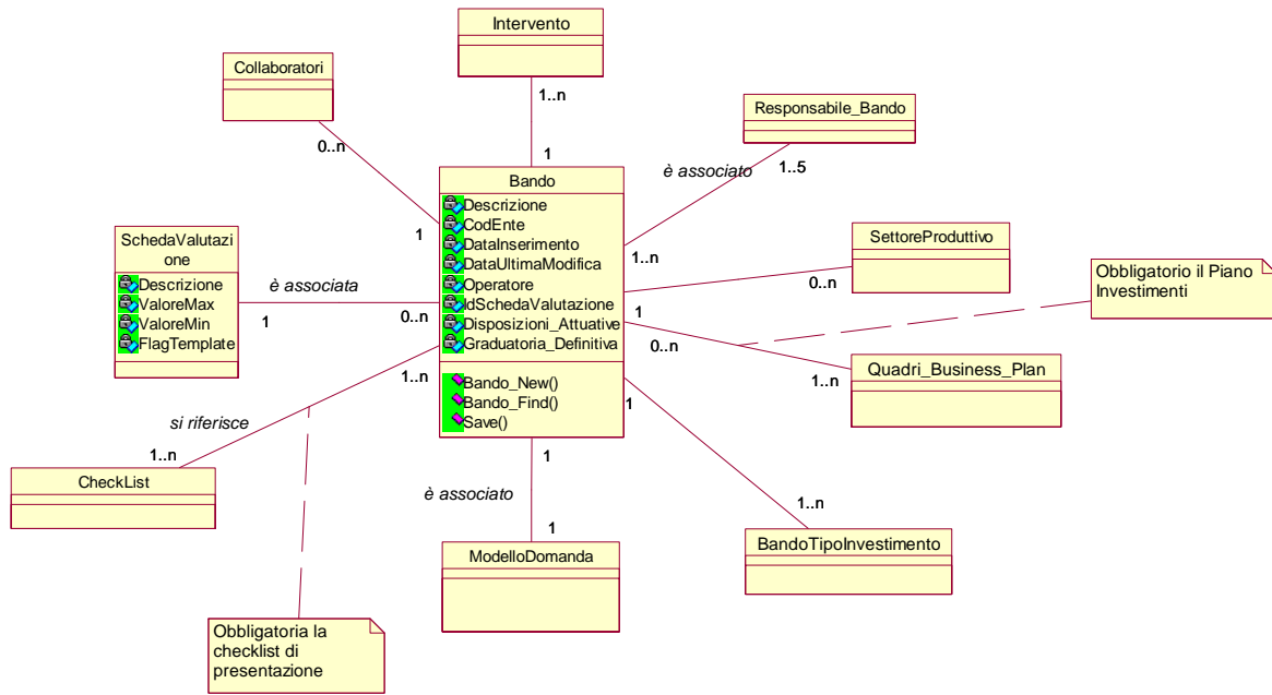
FIGURA 2 – DIAGRAMMA DELLE CLASSI PER LA PUBBLICAZIONE DEL BANDO
