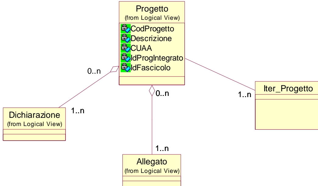
FIGURA 5 – DETTAGLIO PACKAGE PRESENTAZIONE DOMANDA
