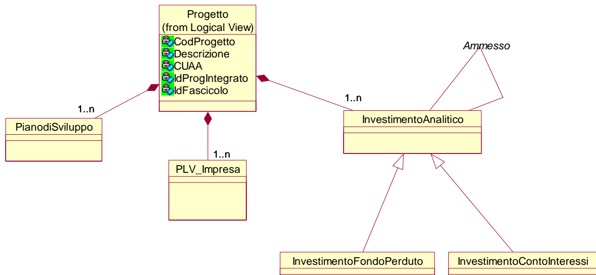
FIGURA 4 – DETTAGLIO PACKAGE BUSINESSPLAN
