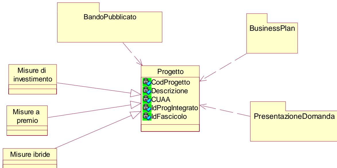
FIGURA 3 – DIAGRAMMA DELLE CLASSI PER IL MODULO PRESENTAZIONE
