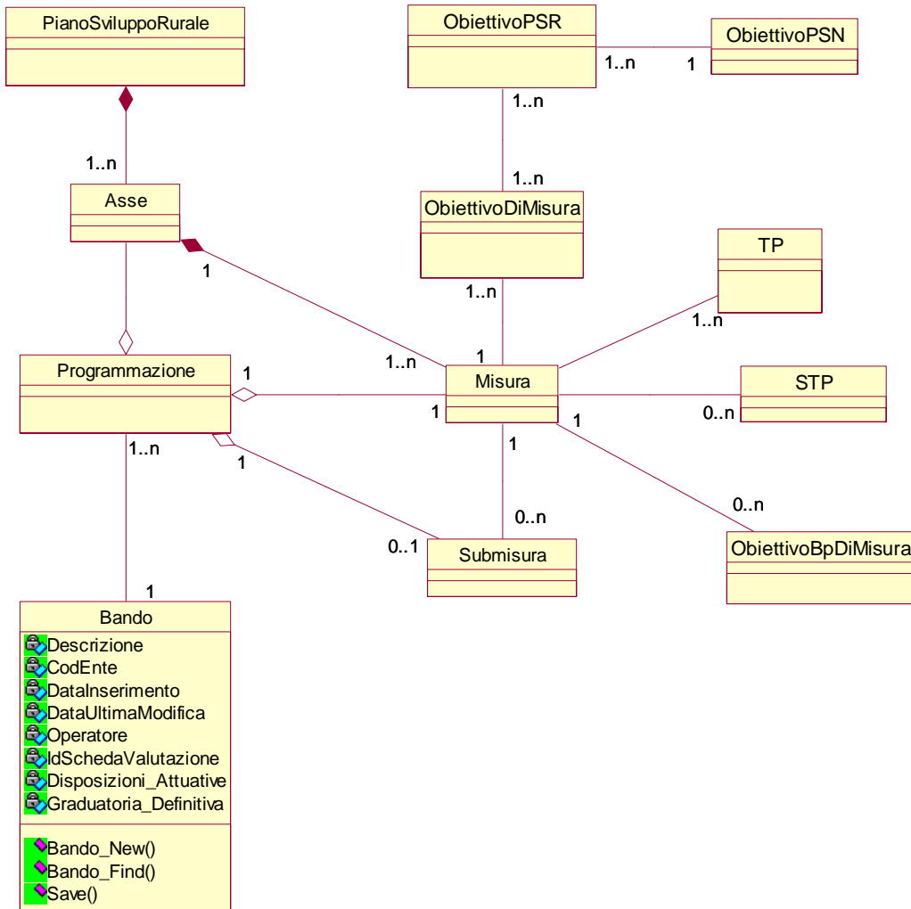
FIGURA 1 - DIAGRAMMA DELLE CLASSI PER IL MODULO DI PROGRAMMAZIONE
