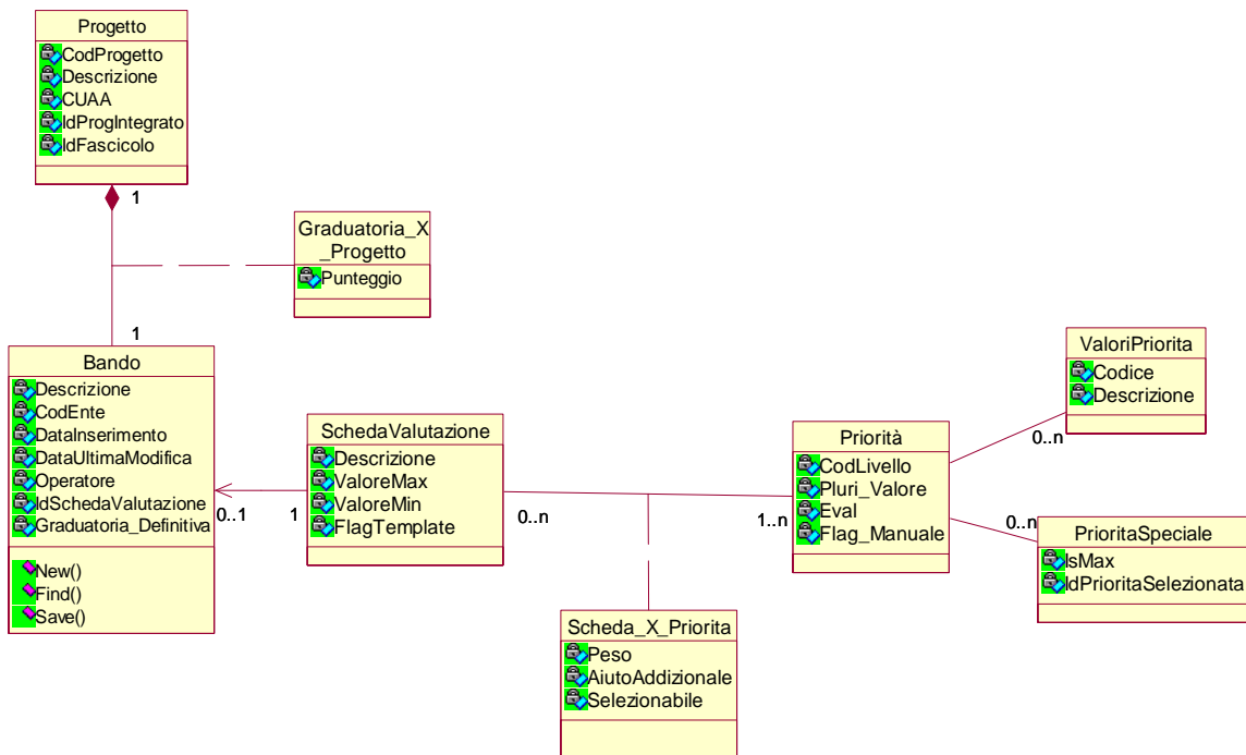
FIGURA 7 – DIAGRAMMA DELLE CLASSI PER IL MODULO VALUTAZIONE
