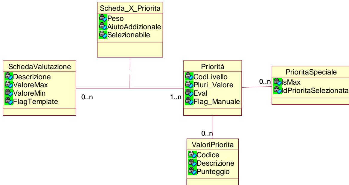
FIGURA 6 – DIAGRAMMA DELLE CLASSI SCHEDA VALUTAZIONE
