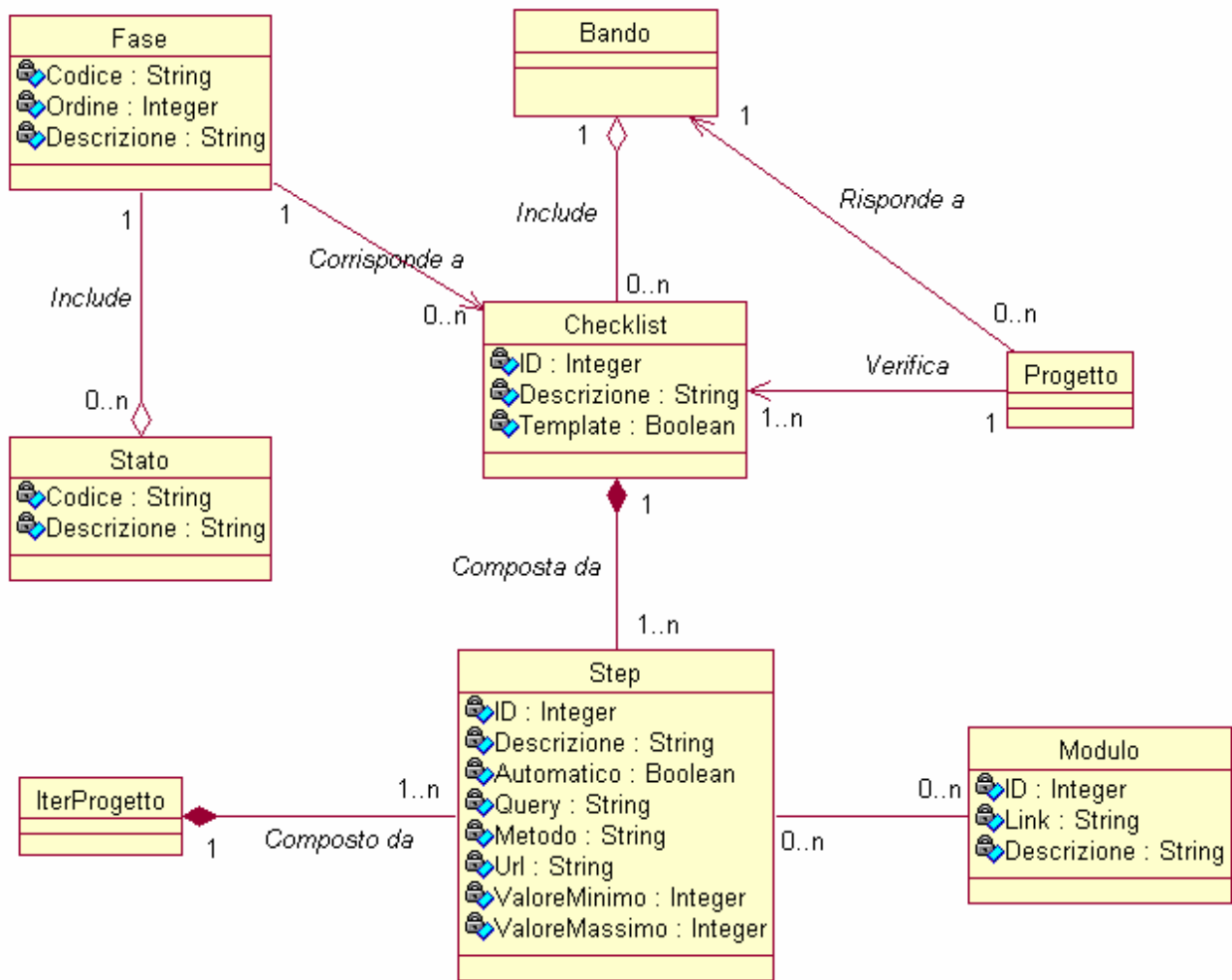
FIGURA 8 – DIAGRAMMA DELLE CLASSI PER IL MODULO PROCEDURALE
